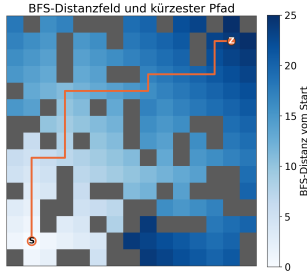
Abbildung 2.4: Breitensuche – Distanzfeld vom Startpunkt und daraus resultierender kürzester Pfad, eigene Darstellung.
