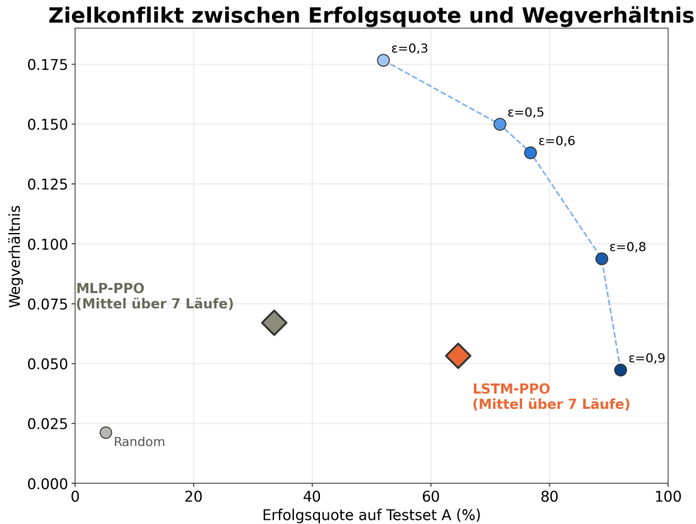
Abbildung 5.6: Evaluation – Erfolgsquote gegen Wegverhältnis für alle Verfahren, eigene Darstellung.
