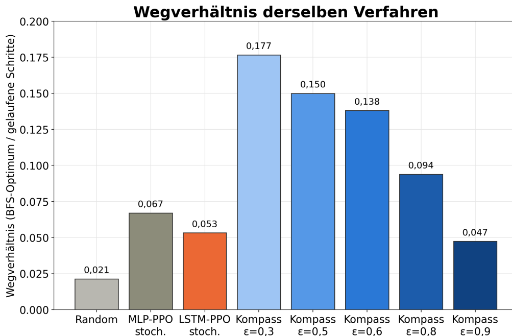
Abbildung 5.3: Evaluation – Wegverhältnis der Verfahren in derselben Achsenordnung, eigene Darstellung.
